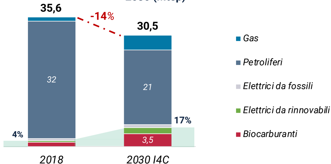
Consumi energetici del settore dei trasporti per fonte nel 2018 e nel 2030 (Mtep)
