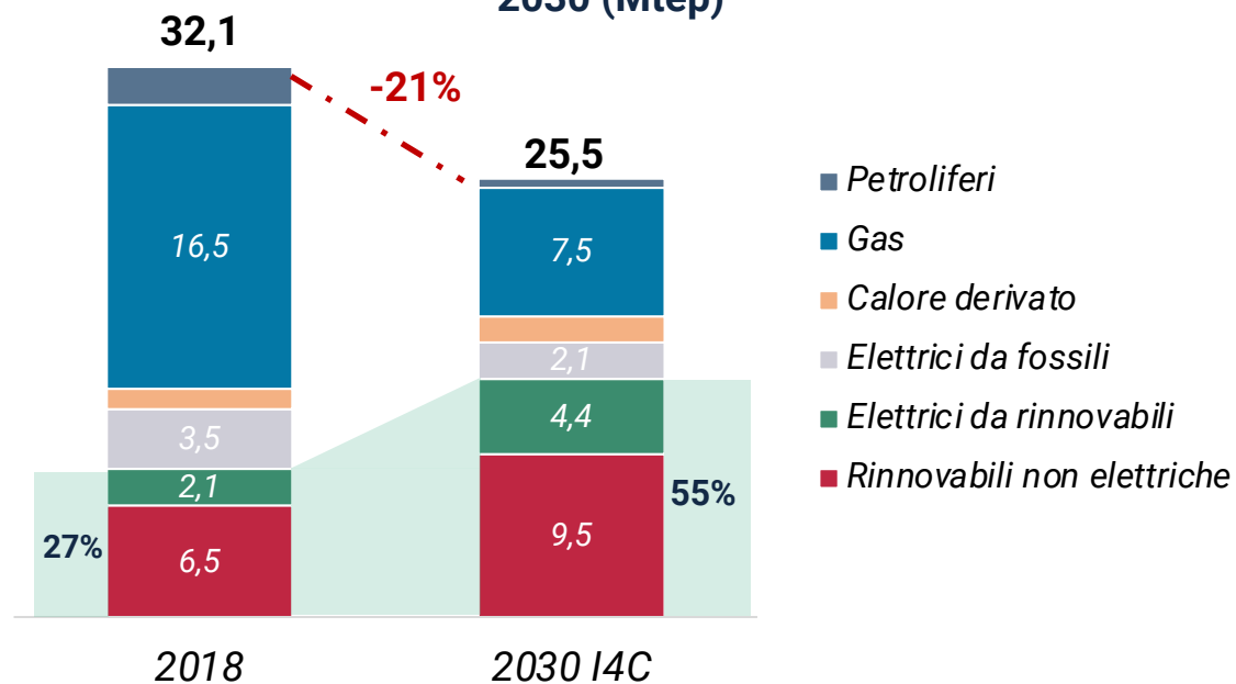
Consumi energetici del settore residenziale per fonte nel 2018 e nel 2030 (Mtep)
