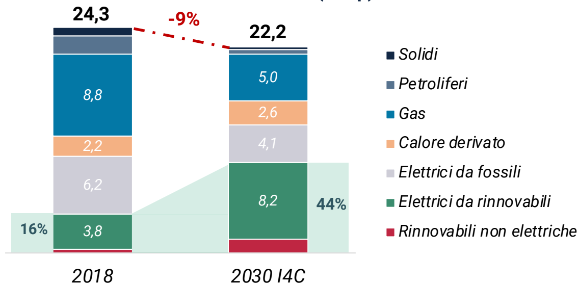
Consumi energetici del settore industriale per fonte nel 2018 e nel 2030 (Mtep)
